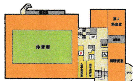
2階
